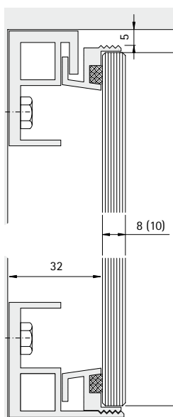
Standardbefestigungssystem
