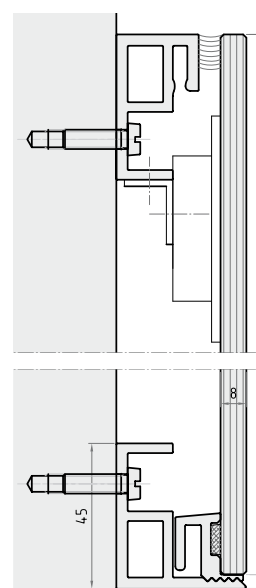
Magnetbefestigungssystem
